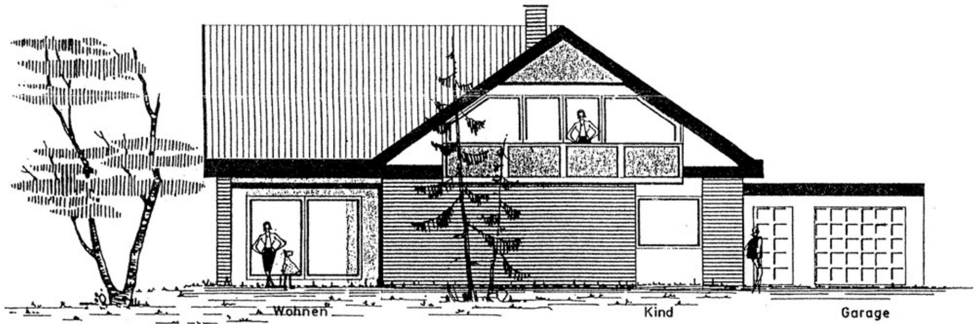
Ansicht - Süd
